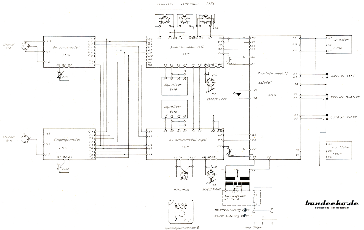
Blockschaltbild mixer 1222
