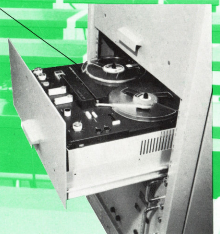
Tragbares Tonbandgerät für zentrale Programmübertragung und Einsatz in den Klassen in TE 100 .
