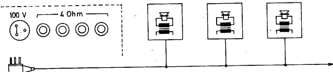
100 V Lautsprecheranpassung
