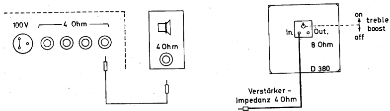
1 Lautsprecherbox D 380
