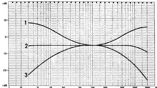
Bild 5 Frequenzgang nach Abs. 2.8.3
