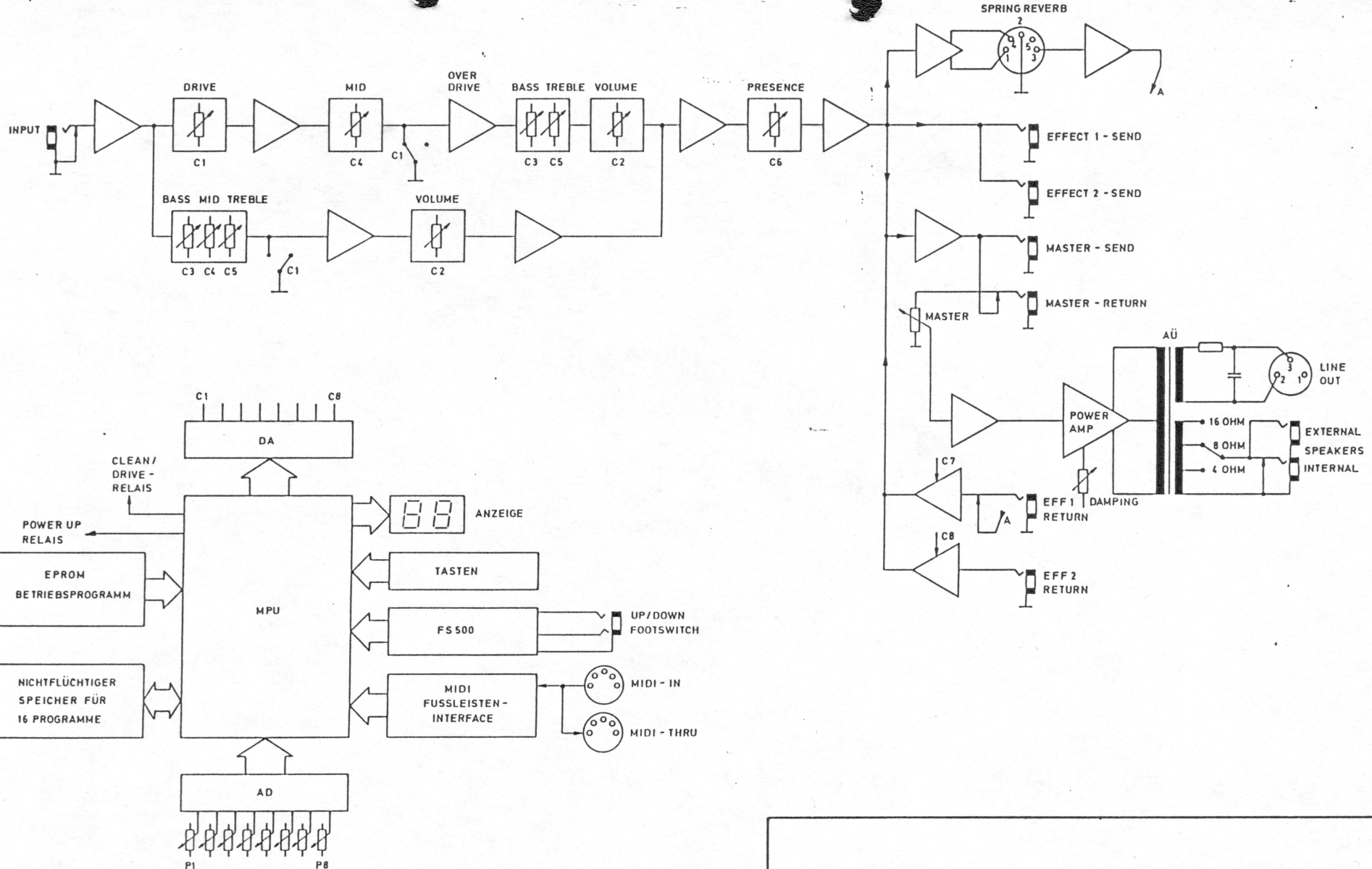
Blockschaltbild 334 274 Reference 500 / 1000 3.
